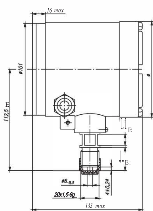
Рисунок Б - Габаритные и присоединительные размеры приборов
