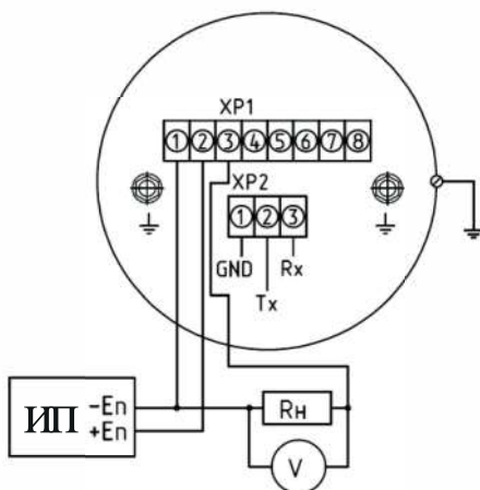
Рисунок В.2 - Прибор ДМ5002Вн-Б
