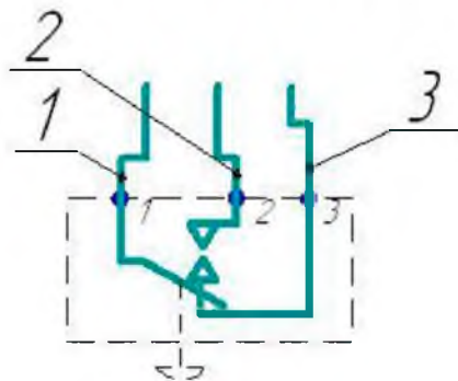
Датчик-реле перепада напора ДЕ 57-2,5ПН
