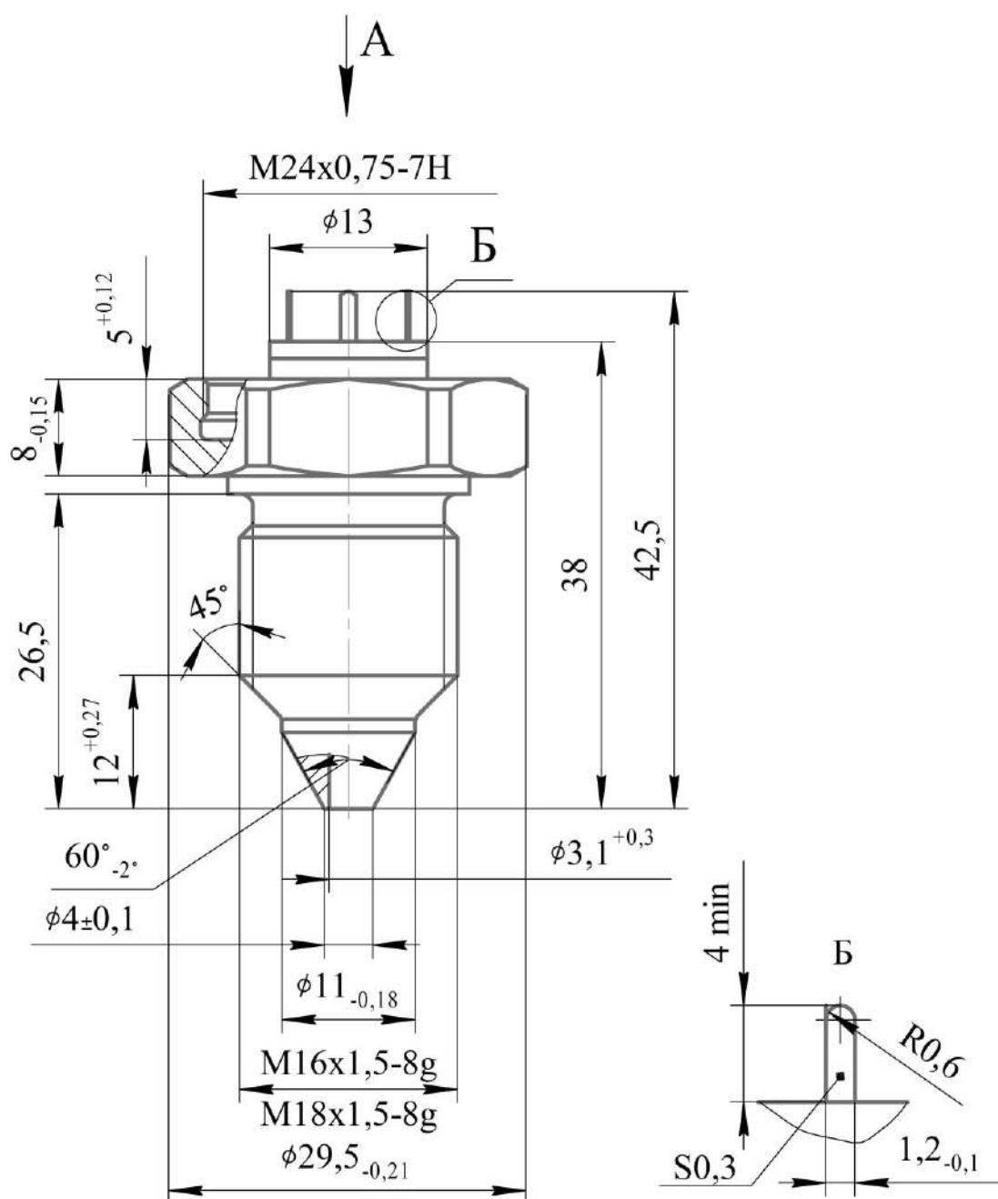
Рисунок Б.1 – HD 100(160...500)-...-MH1(MH2)-P
