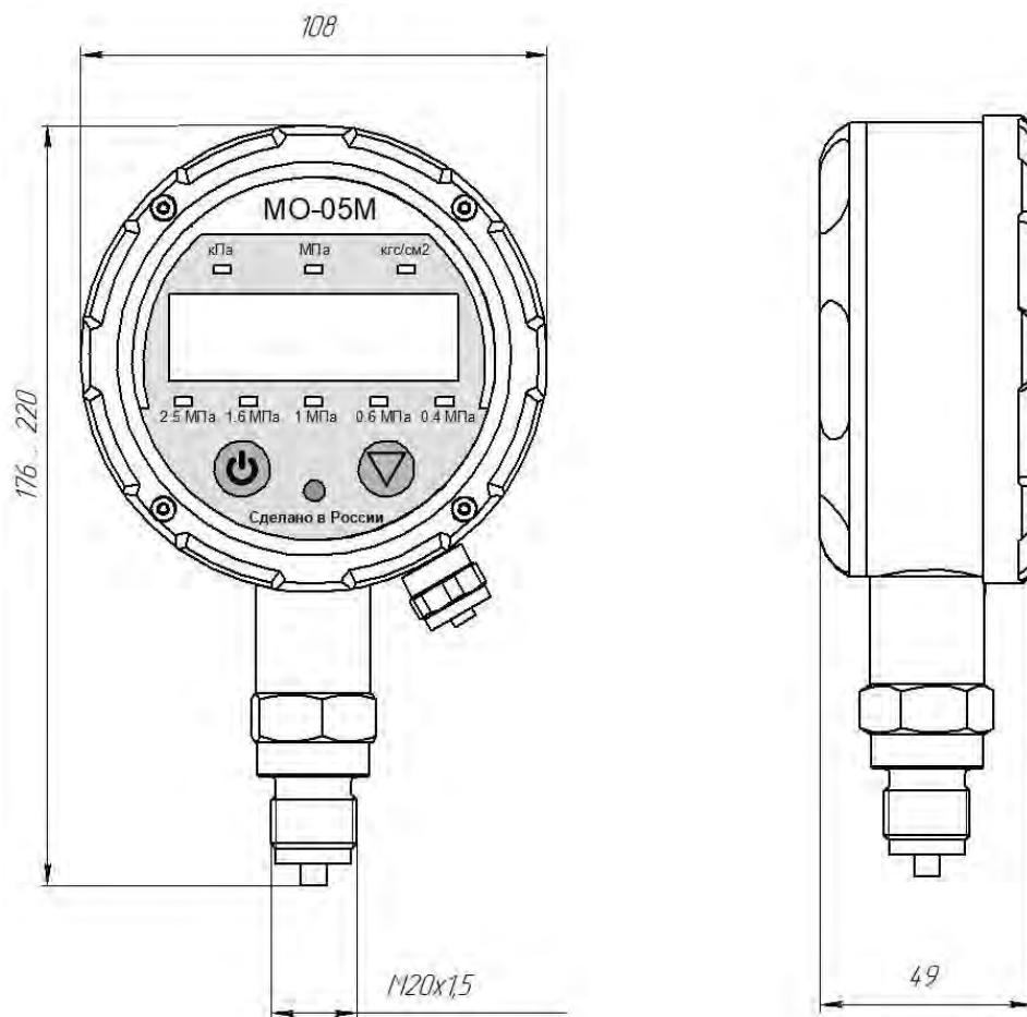
Рисунок 3 – манометры с не съемной ИГ и СДИ дисплеем (исполнение 3).
