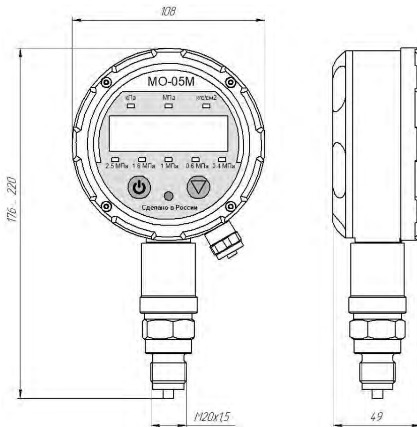
Рисунок 1 – манометры со съемной ИГ (крепление типа накидная гайка) и СДИ дисплеем (исполнение 1).
