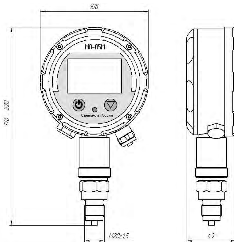
Рисунок 5 – манометры со съемной ИГ (крепление типа накидная гайка) и ЖК дисплеем (исполнения 5 и 8). Внешний модуль МС устанавливается на исполнения 5МС и 8МС.
