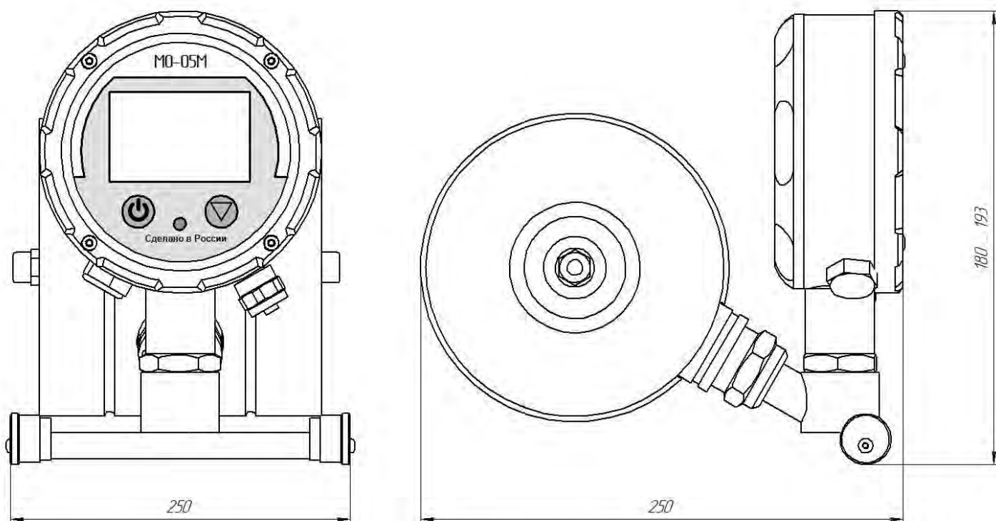
Рисунок 4 – манометры с не съемной ИГ типа «Улитка» и ЖК дисплеем (исполнение 4). Внешний модуль МС устанавливается на исполнение 4МС.
