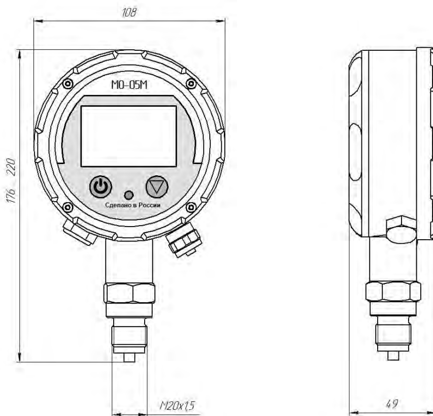
Рисунок 6 – манометры с не съемной ИГ и ЖК дисплеем (исполнения 6 и 7). Внешний модуль МС устанавливается на исполнения 6МС и 7МС.
