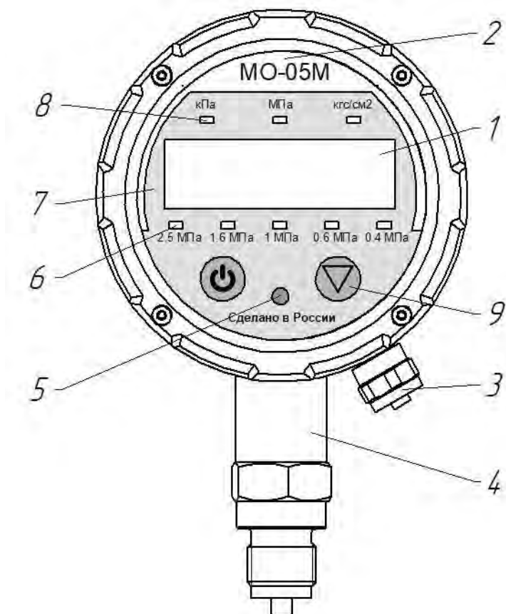
Рисунок 1. Внешний вид МО-05М с СДИ дисплеем и не съемной ИГ
