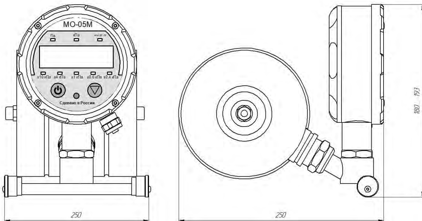
Рисунок 2 – манометры с не съемной ИГ типа «Улитка» и СДИ дисплеем (исполнение 2).
