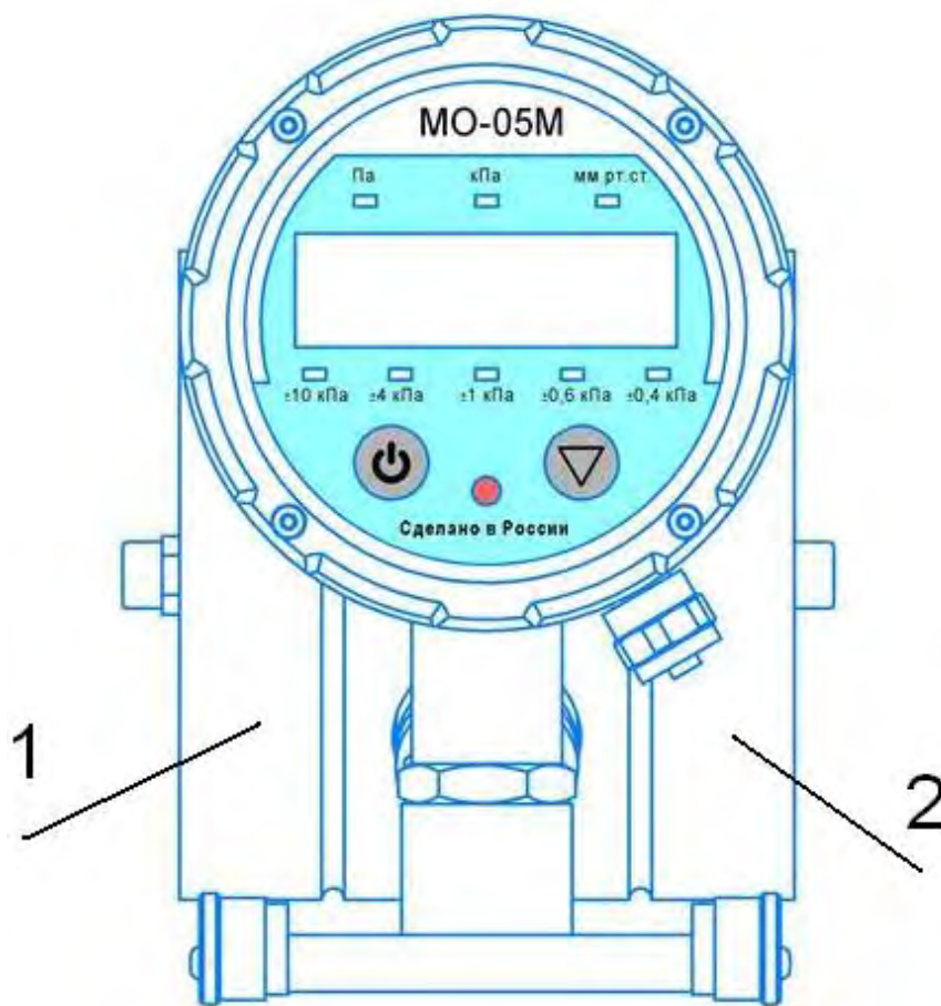
Рисунок 4. Внешний вид МО-05М с ИГ типа «улитка» с СДИ дисплеем
