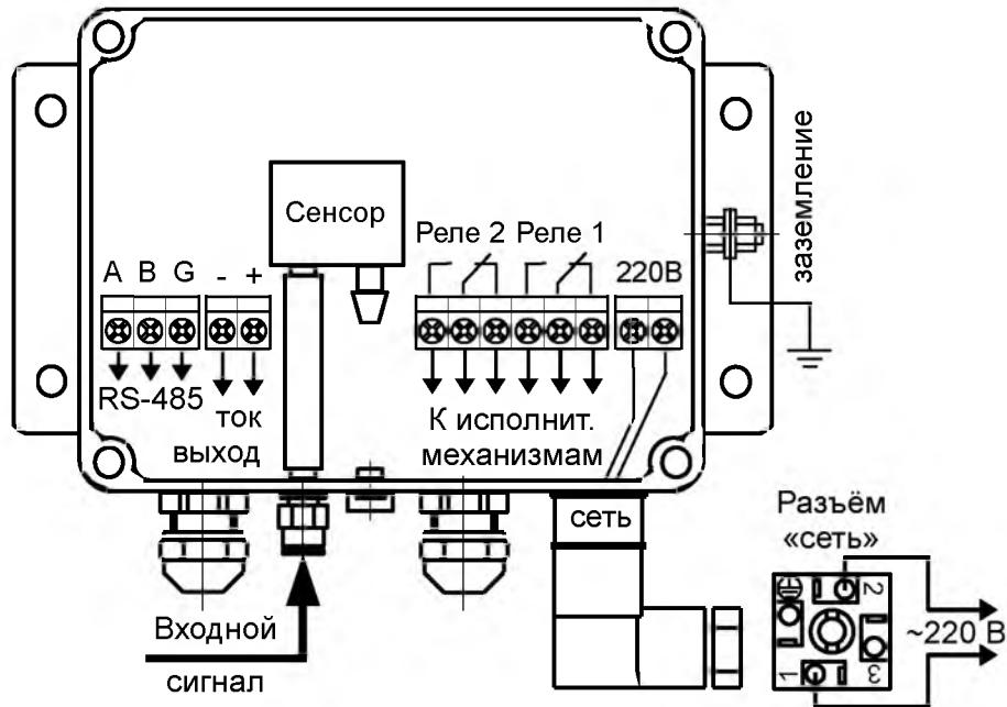
Рисунок Г.3 - Внешние соединения прибора настенного исполнения ПКД-1115.Т, ПКД-1115.Н, ПКД-1115.ТН (крышка снята)
