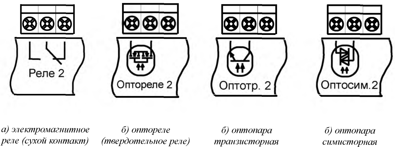
Рисунок В.2 - Маркировка дискретных выходов прибора настенного исполнения
