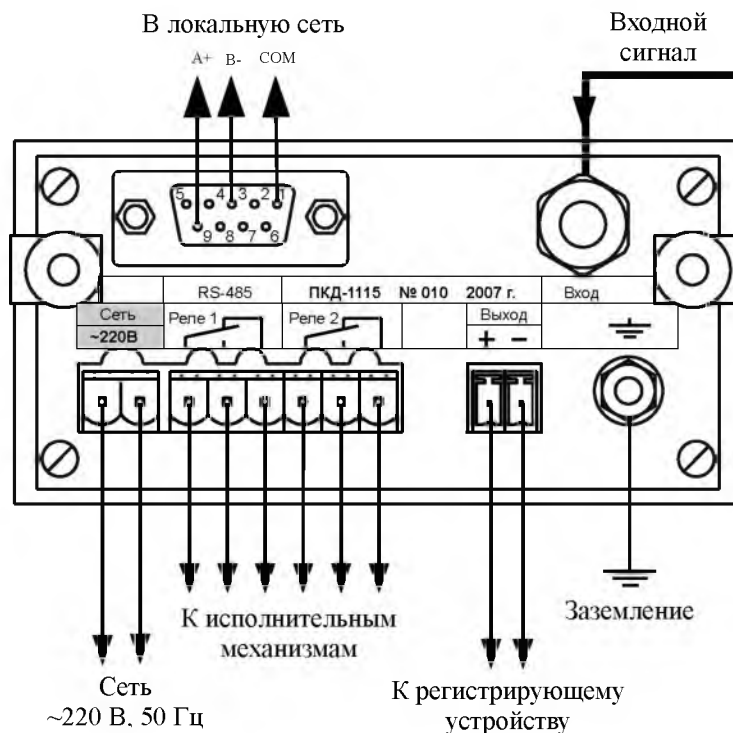
Рисунок Г.1 - Внешние соединения приборов щитового исполнения ПКД-1115.Т, ПКД-1115.Н, ПКД-1115.ТН
