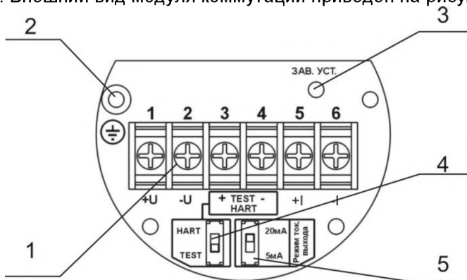
Рисунок 2.3 — Модуль коммутации
